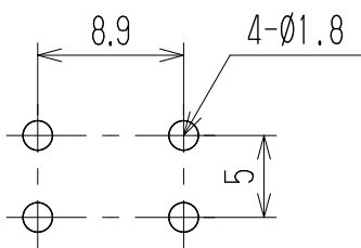
基板取付穴参考図
